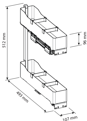
ESPECIERO EXTRAÍBLE 150 mm
