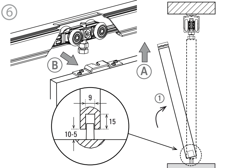
Pletina lateral DN50/80 Pletina lateral DN50/80 Lateral door bracket DN50/80
