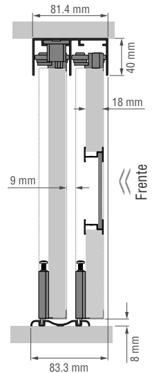
Vista Lateral
