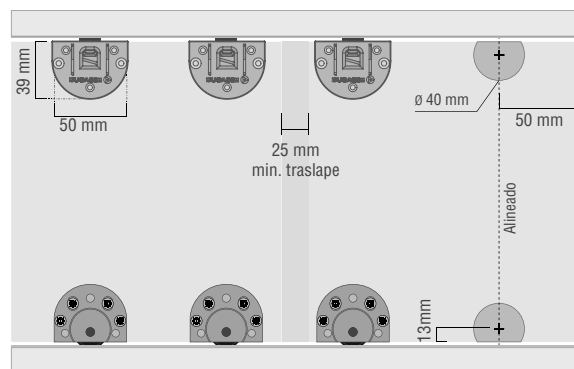
Vista Posterior
