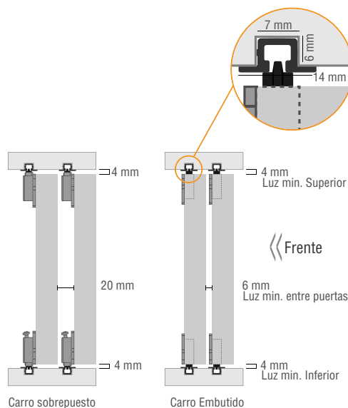
Vista Lateral
