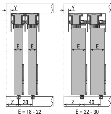
Riel Embutido CX Triho Embutido CX Inlaid Carrier Track CX
