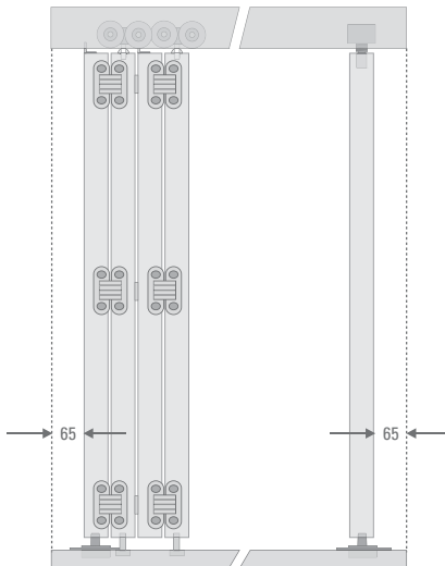
Vista frontal sistema plegado
