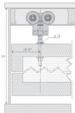
Vista Frontal Montaje sin placa + Guía Simple 35
