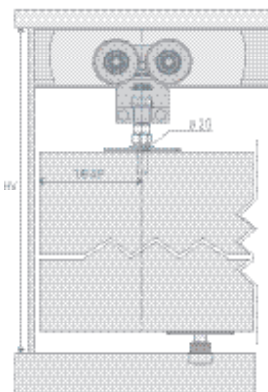
Vista Frontal Montaje con placa + Guía PG 35
