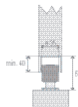
Aplicación con Guía PG 35 (accesorio)
