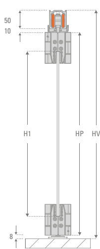
Vista Lateral Puertas plegadas:
