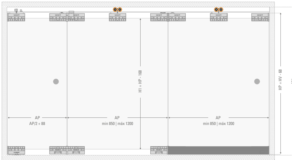
KIT 2H TAURO PLVD80 ANG + KIT COMPLEMENTO TAURO CENTRO VD
