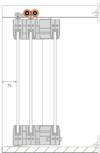
Vista Frontal Puertas plegadas:
